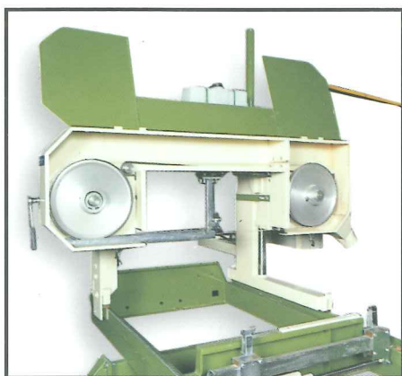
Timber Queen S Sägekopf mit offener Tür
