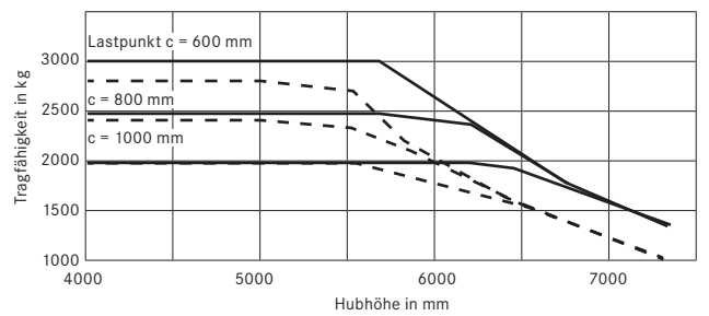
Tragfähigkeiten RX 60-30/600 mit Dreifach-Hubgerüst
