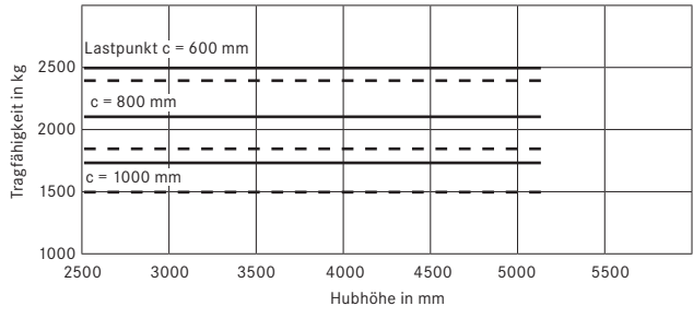
Tragfähigkeiten RX 60-25/600 Tele-/Niho-Hubgerüst
