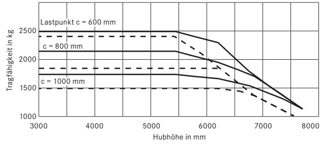
Tragfähigkeiten RX 60-25/600 mit Dreifach-Hubgerüst
