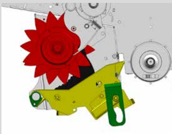
Fond mouvant en position de travail.
