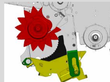
Fond mouvant en position entièrement abaissée.
