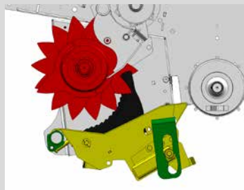
Fond mouvant en position intermédiaire.
