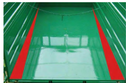
Kipperbrücke in konischer Bauweise, vorne 2200 mm - hinten 2300 mm garantiert ein sicheres Abkippen der Ladung. Spannkette mit Loch und Schraube im ersten Aufsatz (S+SA)
