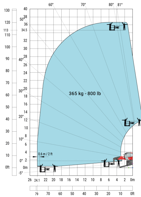
Rotazione su stabilizzatori con cestello da 365 kg
