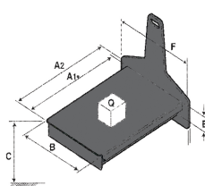
PLF: неподвижная платформа с ящиком
