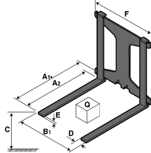
FA: регулируемые вилы
