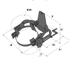
FUT: манипулятор бочек
