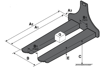
FR: упаковочные вилы
