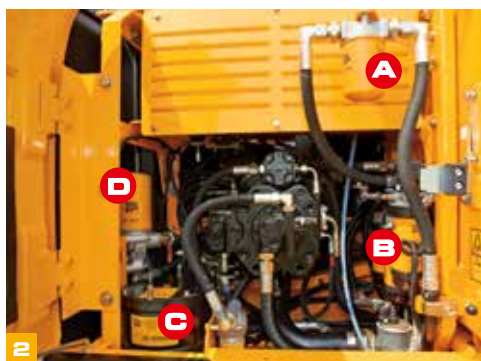
(A) Hydraulikölfilter (B) Kraftstofffilter (C) JCB Plexus-Ölfiltersystem (D) Motorölfilter
