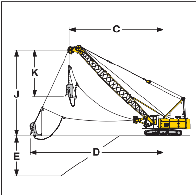
Traglasten in Tonnen (t) für Auslegerlängen von 11 m bis 26 m Ballast 16.4 t
