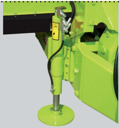
Hydraulischer Stützfuß mit Bedienung über Bordhydraulik Béquille avec commande hydraulique branchée au système hydraulique de la mélangeuse Hydraulische steunpoot verbonden met eigen hydraulisch systeem
