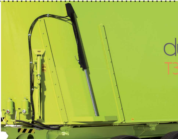
Seitenschieber für Direktaustrag Trappe de déchargement direct Directe losdeuren
