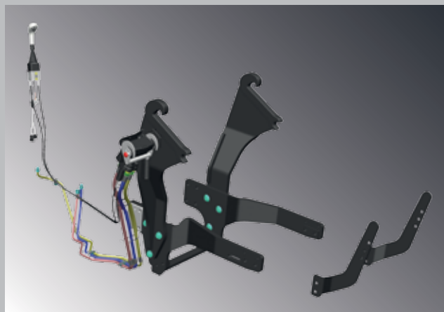
Conjuntos de preinstalación para pala cargadora de fábrica. La elección es suya.
