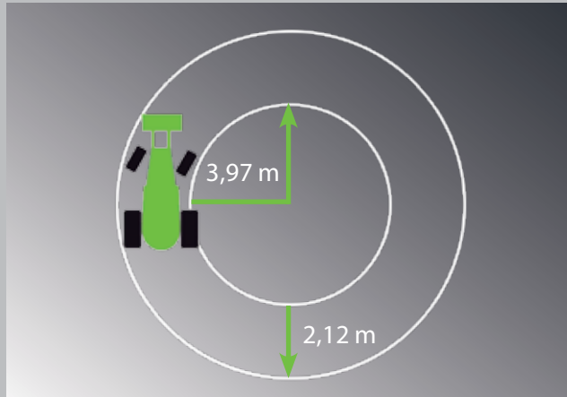
Un radio de giro de 3,97 m permite maniobrar con facilidad incluso en los espacios más reducidos (en función de los neumáticos y el entorno).
