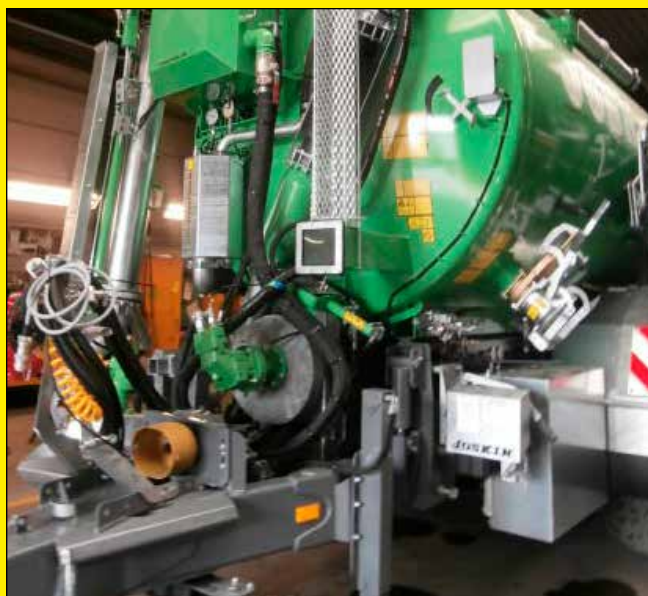
STORM con accionamiento hidráulico Power-Pack
